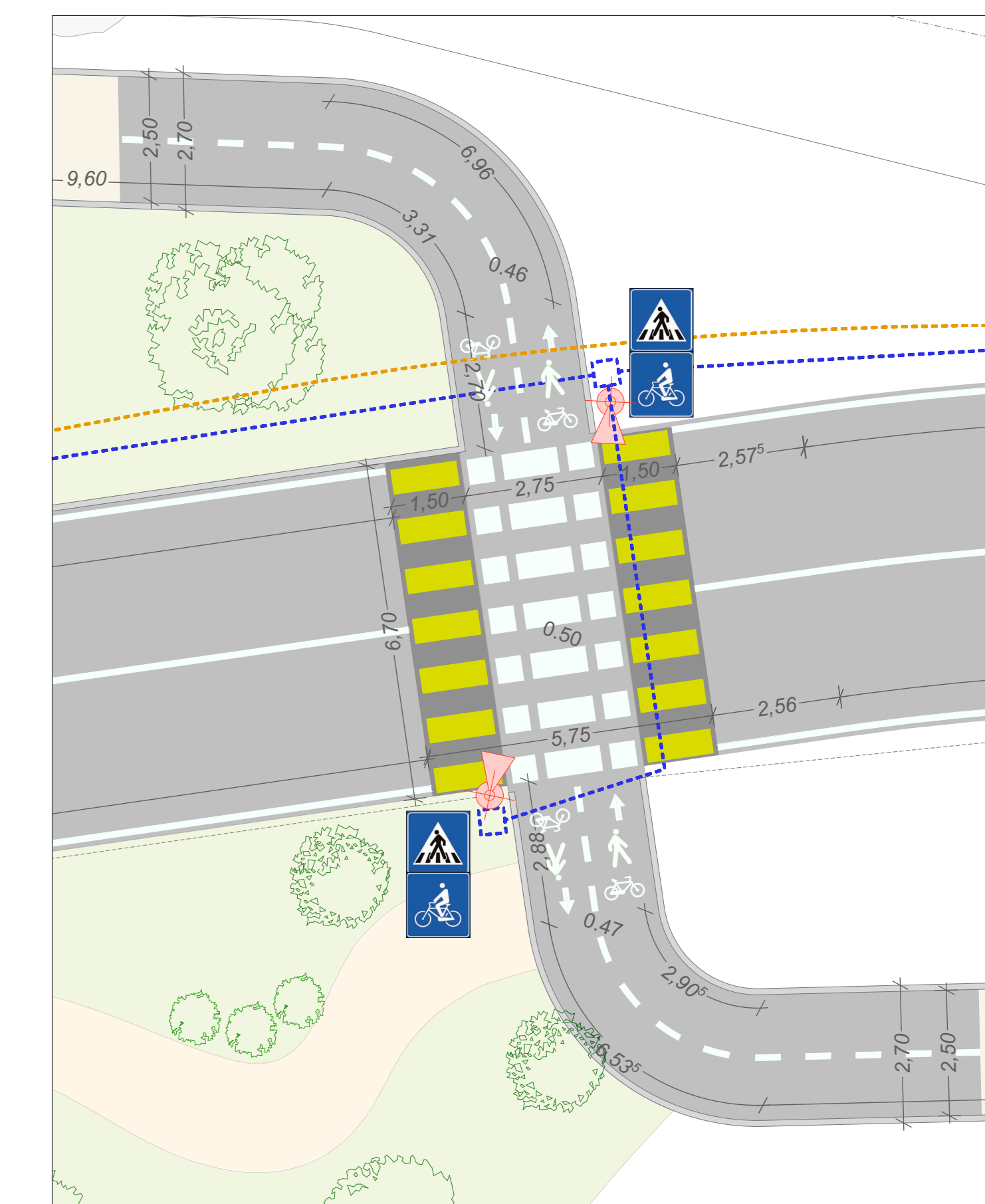
DETTAGLIO ATTRAVERSAMENTO PEDONALE - 1: 100
