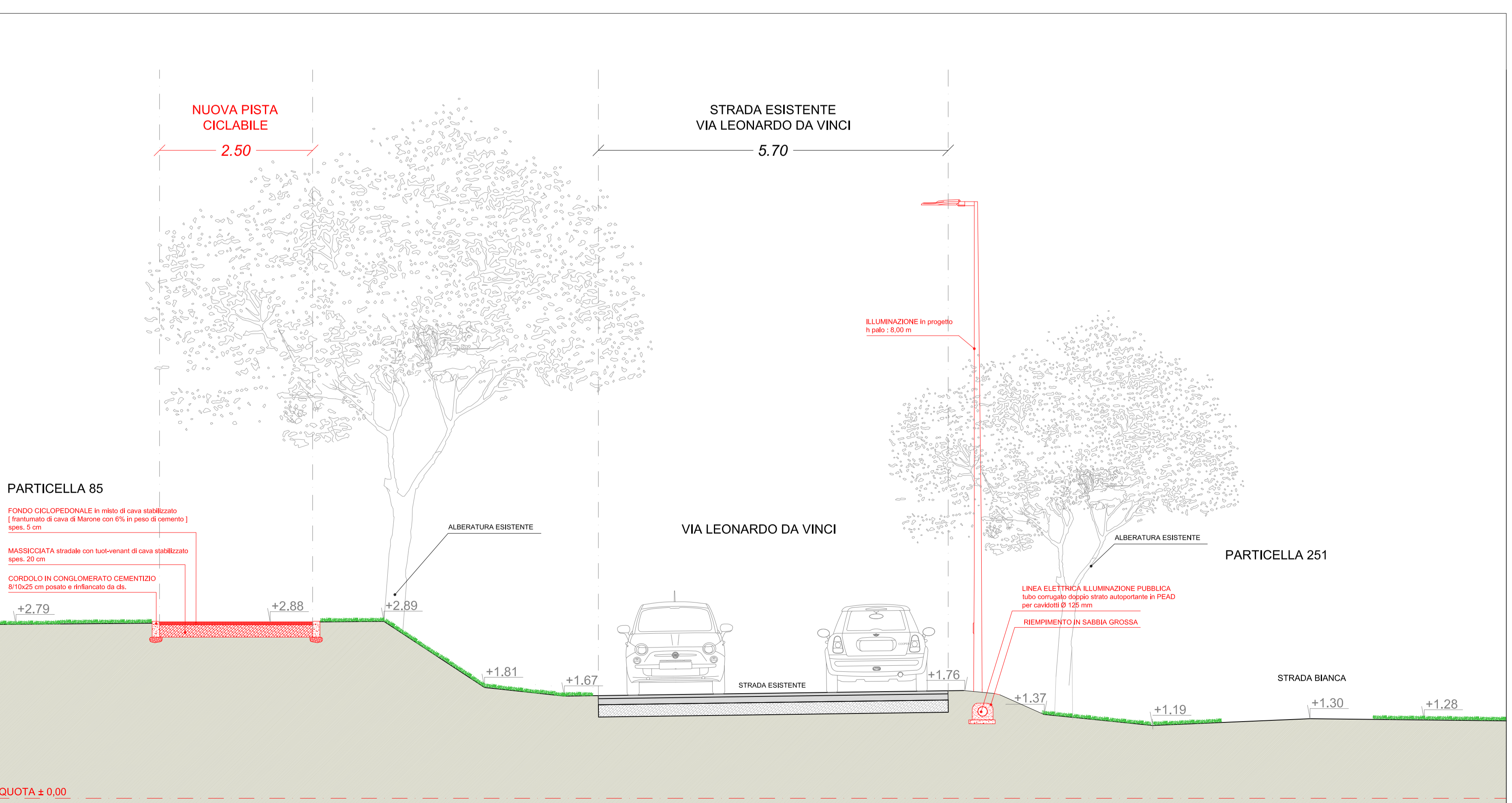
SEZIONE A/A - RAFFRONTO
