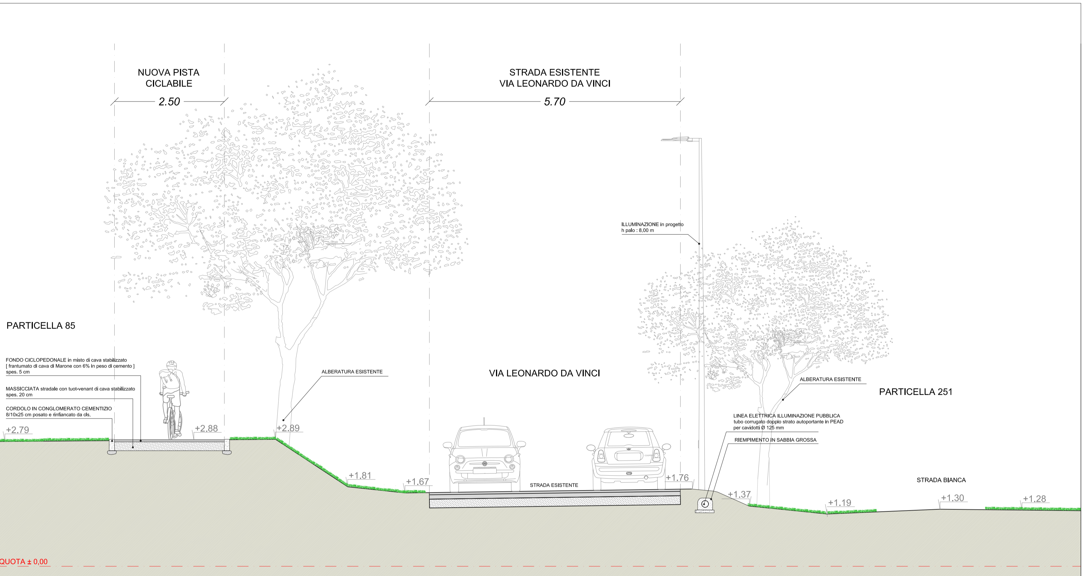
SEZIONE A/A - PROGETTO
