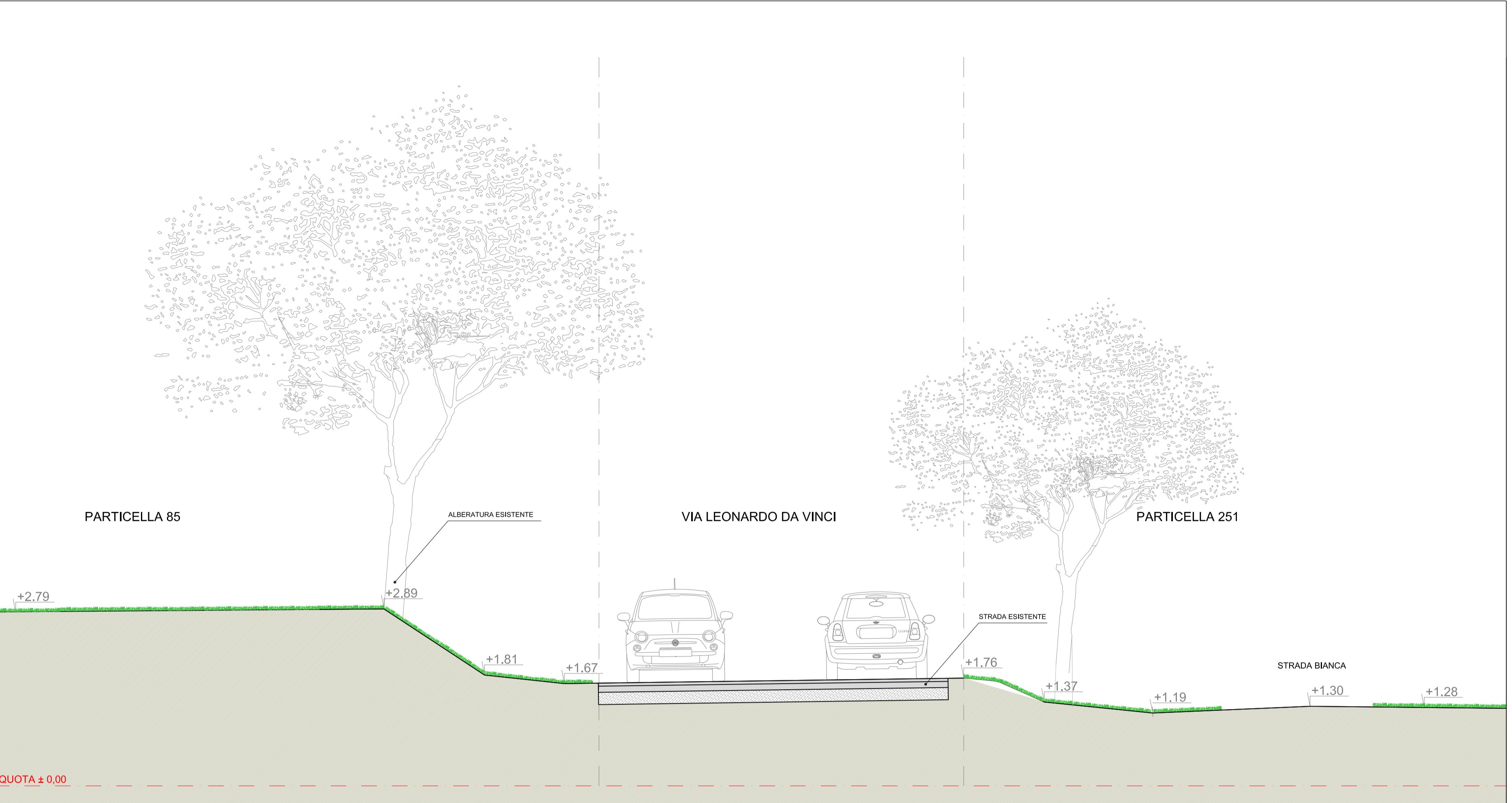
SEZIONE A/A - STATO DI FATTO
