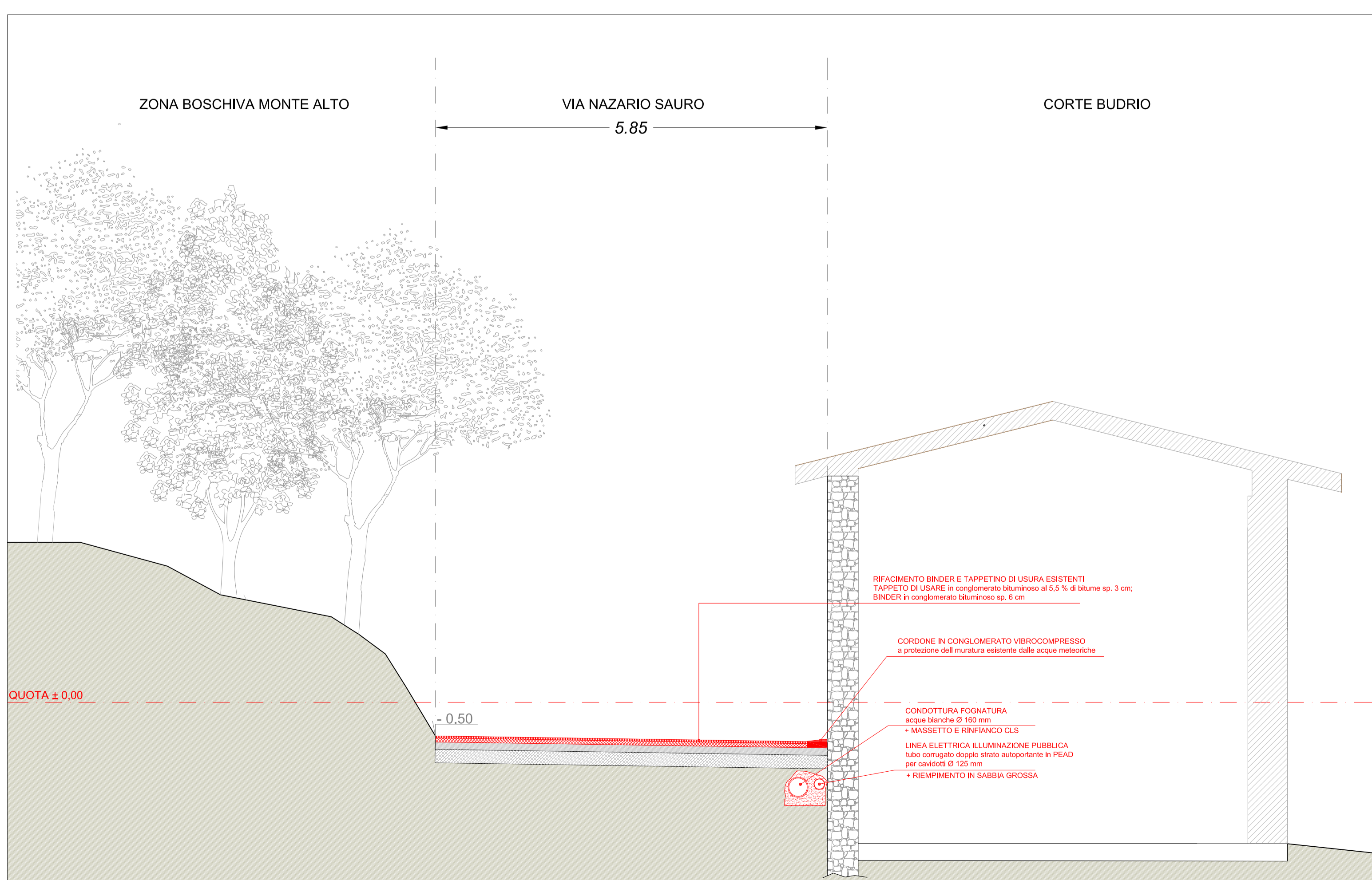
SEZIONE D/D - RAFFRONTO
