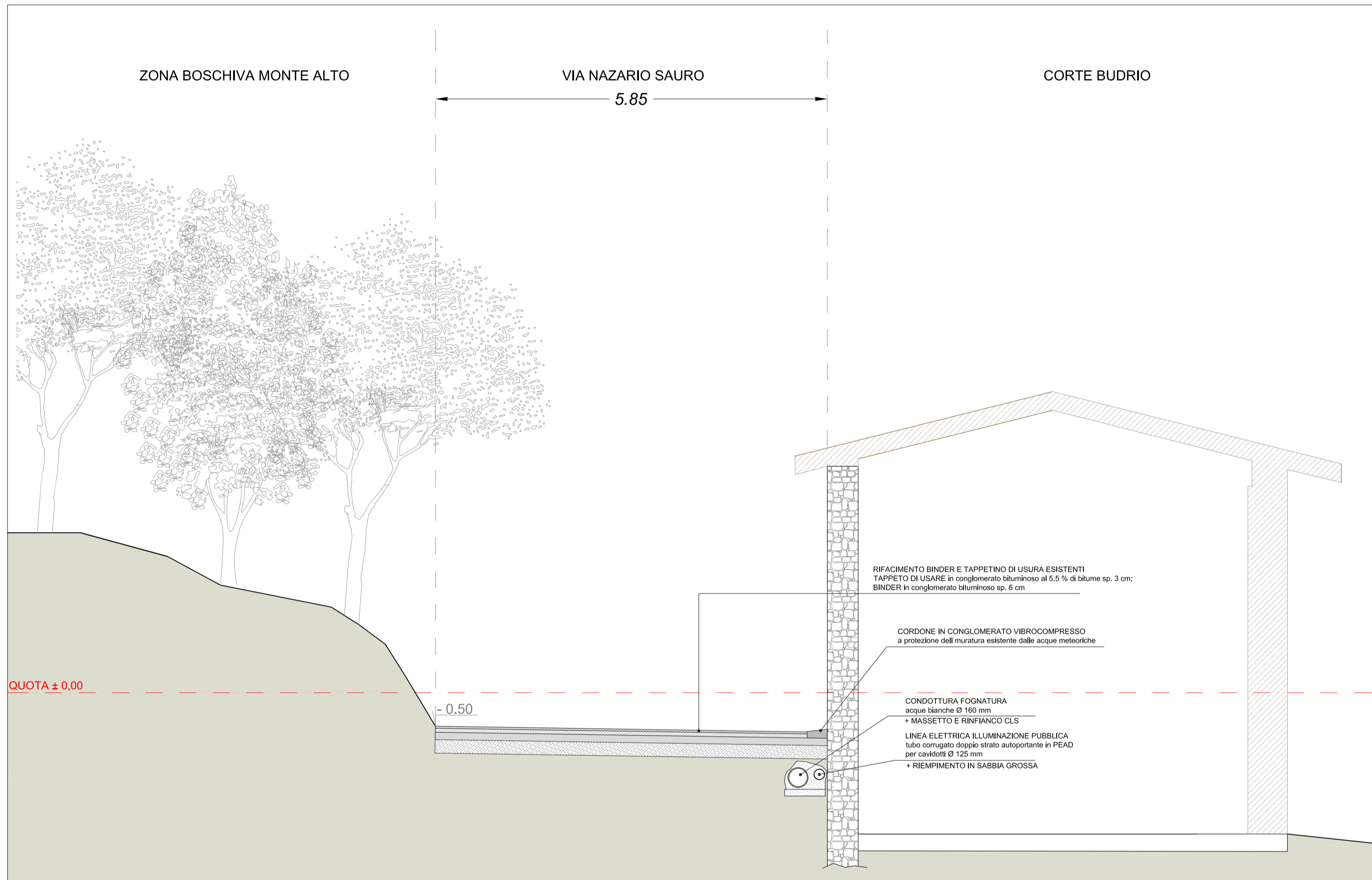
SEZIONE D/D - PROGETTO
