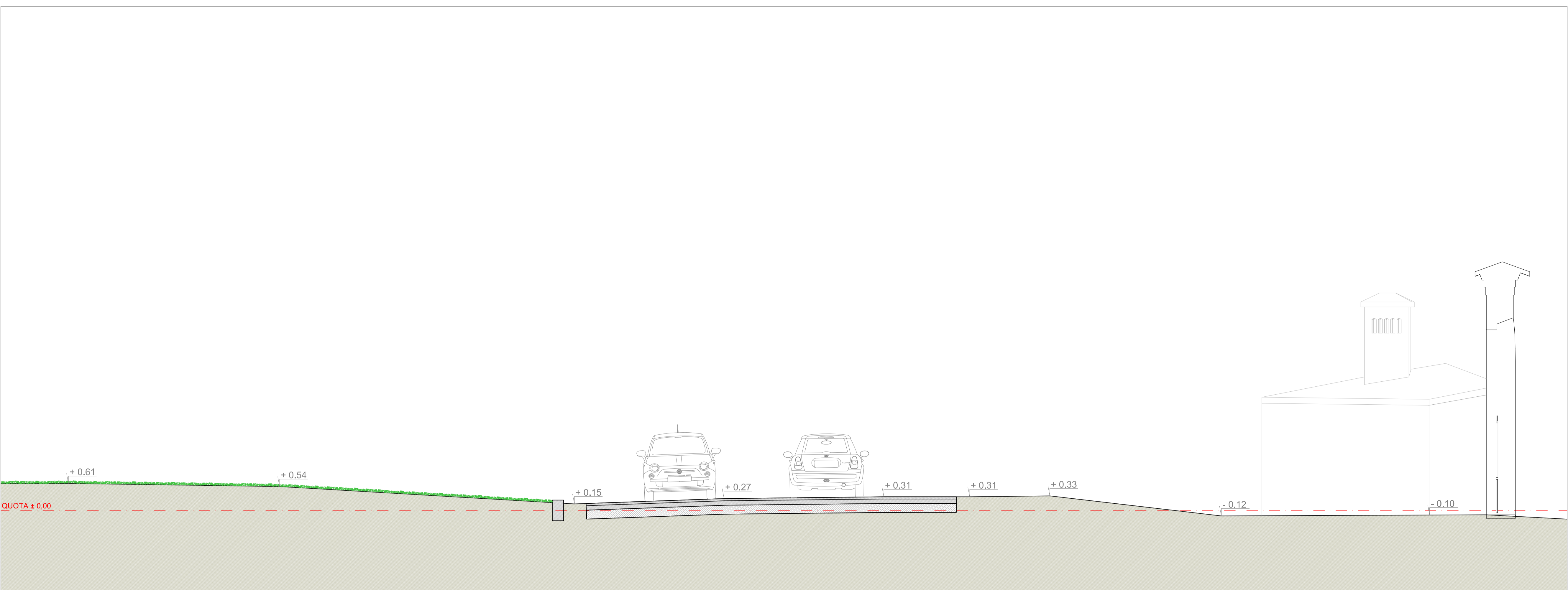
SEZIONE C/C - STATO DI FATTO
