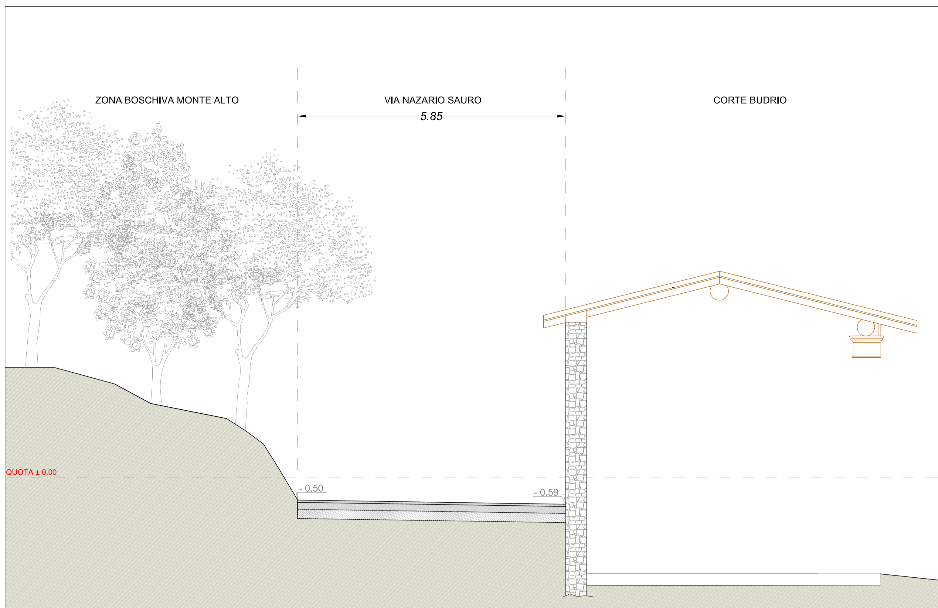
SEZIONE D/D - STATO DI FATTO
