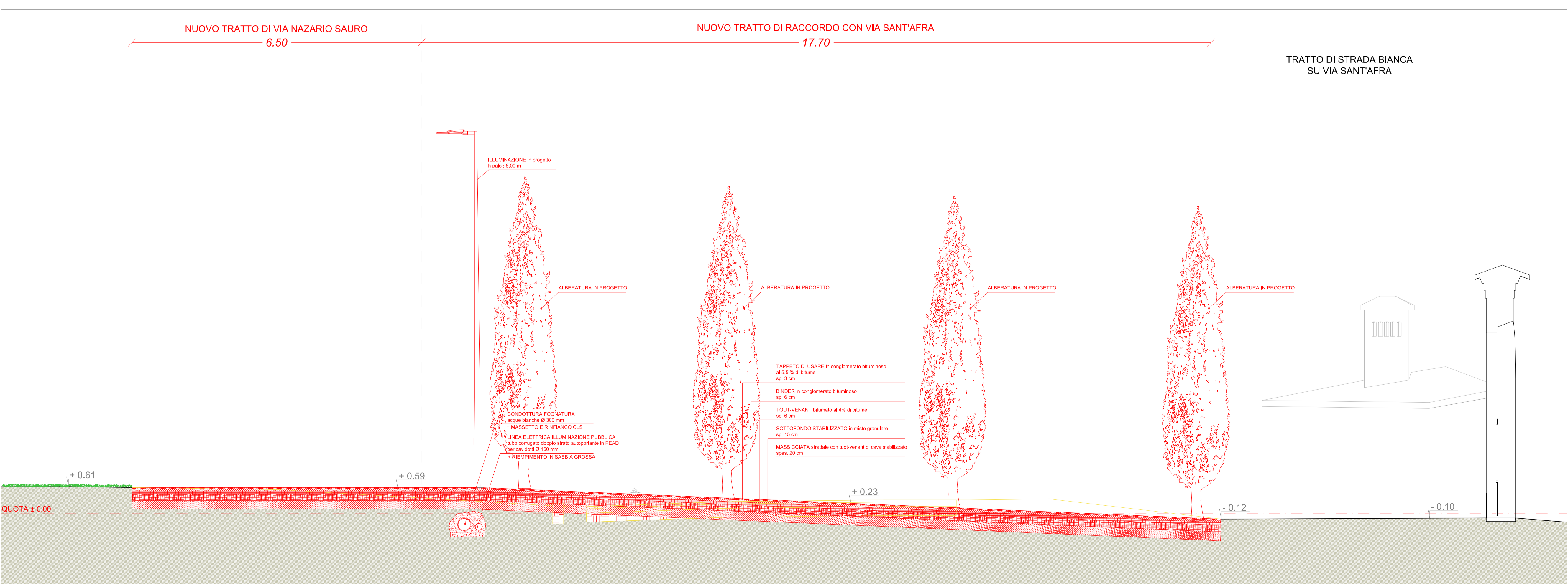
SEZIONE C/C - PROGETTO
